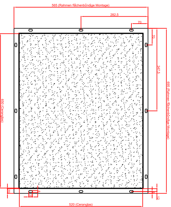
Ausschnitt in Abdeckung flächenbündiger Einbau 656mm x 526mm
