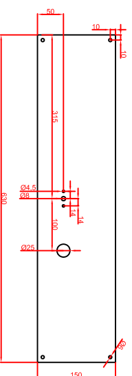
Schalterblende (optional lieferbar)
